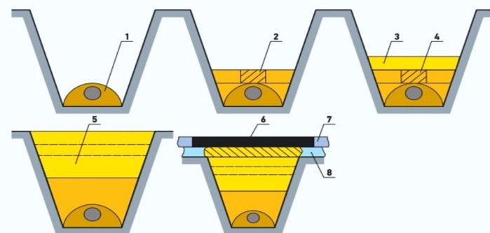
Рис. 1. Типовая технологическая схема обратной засыпки самотечного трубопровода водоотведения из ТПСС (а — подбивка грунта под трубу штыками, б — засыпка и уплотнение песка в пазах электротрамбовками и в защитной зоне на 30 см выше труб вручную, в — засыпка и уплотнение песка на 75 см выше труб ручными инструментами-электротрамбовками (виброплитами до 50 кг), г — засыпка песка верхней зоны траншеи и уплотнение виброплитами до 100 кг, д — восстановление дорожного основания и покрытия дороги; 1 — трубопровод в траншее; 2 — засыпка песком пазух и защитной зоны; 3 — засыпка песка выше трубопровода на 70 см; 4 — защитный слой песка; 5 — окончательная засыпка; 6 — уплотнение и восстановление работ; 7 — восстановление дороги; 8 — окончательная засыпка).
